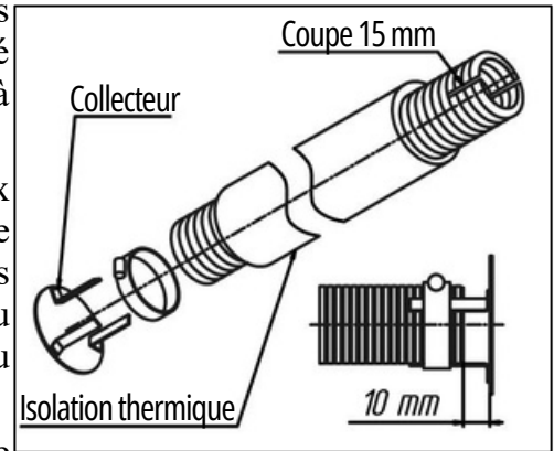
Fig. 9 - Collecteur du tuyau d'échappement
