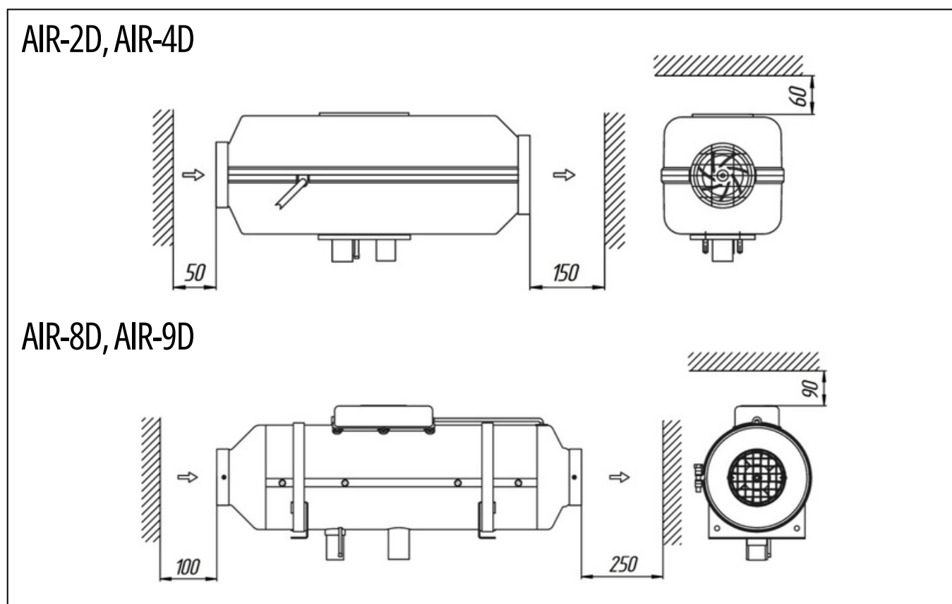
Fig.1b - Distances des parois
