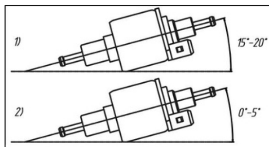
Fig. 18 - Angle d'installation de la pompe à carburant TH-9; TH-10; TH-11 (1) et de la pompe à carburant Thomas Magnete (2).
