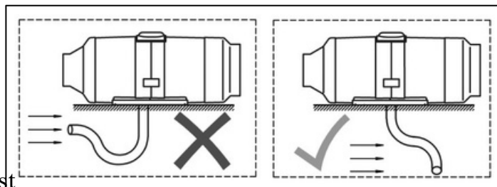
Fig. 5 - Position du tuyau d'admission d'air /
