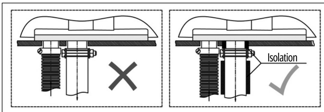
Fig.12 - Installation d'une isolation thermique supplémentaire
