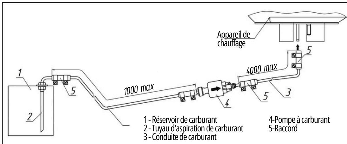
Fig.14 - Exemple d'alimentation en carburant de l'appareil de chauffage avec tuyau d'aspiration de carburant
