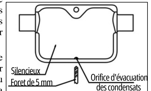
Fig. 10a - Orifice d'évacuation des condensats pour montage horizontal
