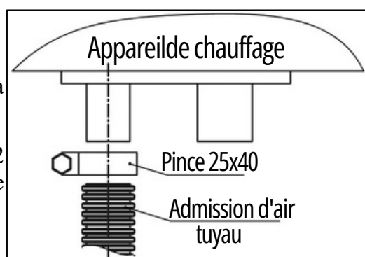
Fig. 4 - Connexion du tuyau d'air à l'appareil
